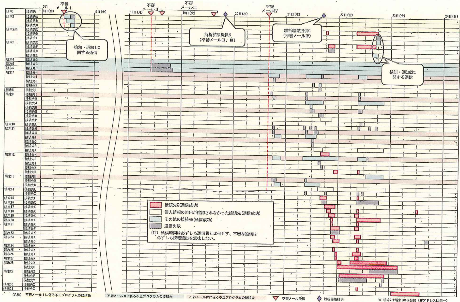
図2 感染端末と不審な通信
